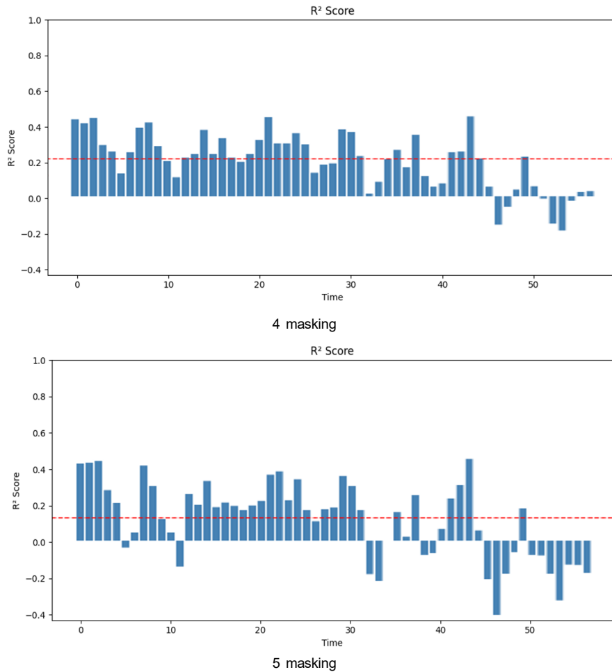
그림 5. 마스킹 수에 따른 성능 비교
