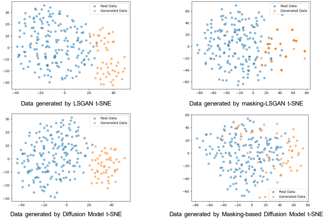
그림 3. 서로 다른 생성 방법에 따라 생성된 데이터와 실제 데이터의 t-SNE 시각화 결과
