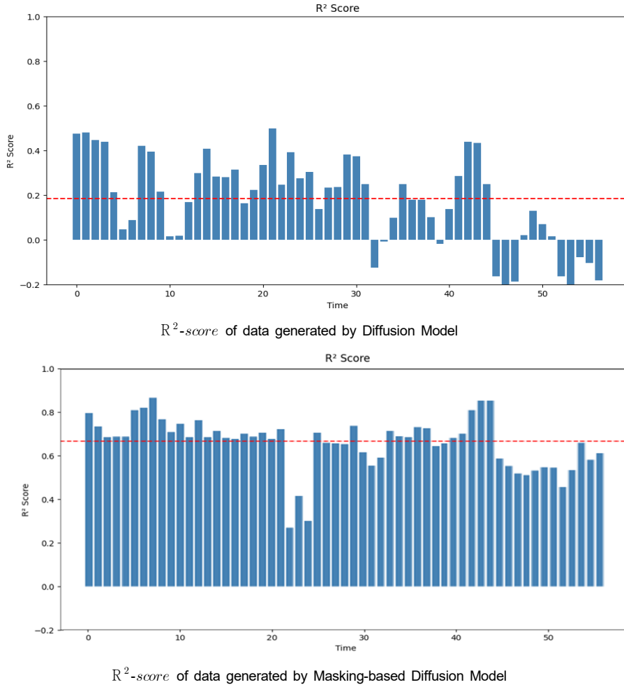
그림 4. 데이터의 R^2 -score
