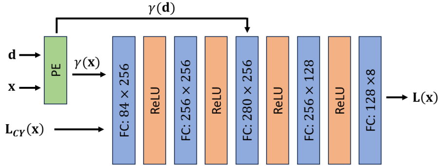
그림 3. 포인트 기반 라디언스 정보 예측기 세부 구조 Fig. 3. Detailed architecture of the point-based radiance predictor
