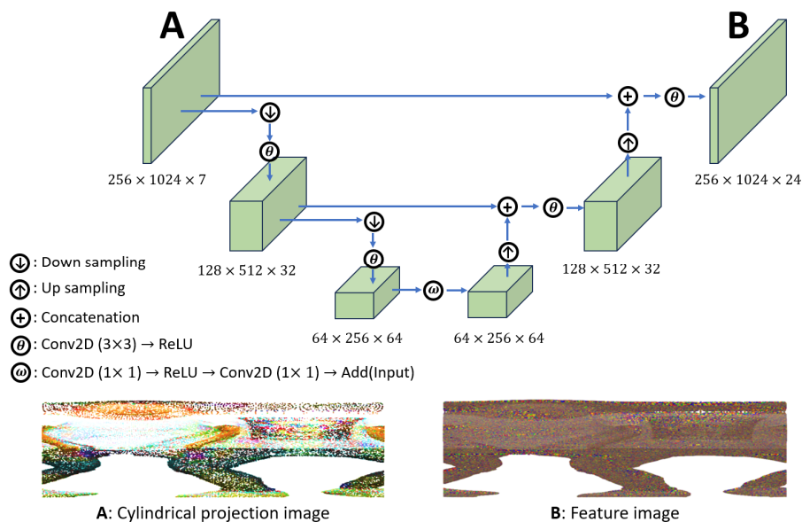
그림 2. 원통형 뉴럴 컨볼루션 네트워크 세부 구조 Fig. 2. Detailed architecture of the cylindrical convolution neural network
